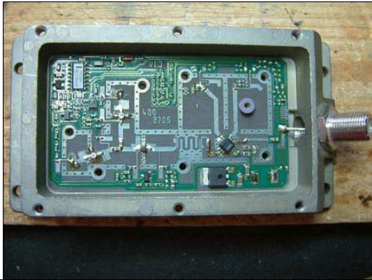
Préparation avant mise en place coaxial
