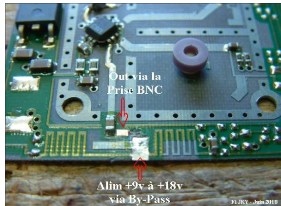
L'OL réglé à 11,100 GHz
